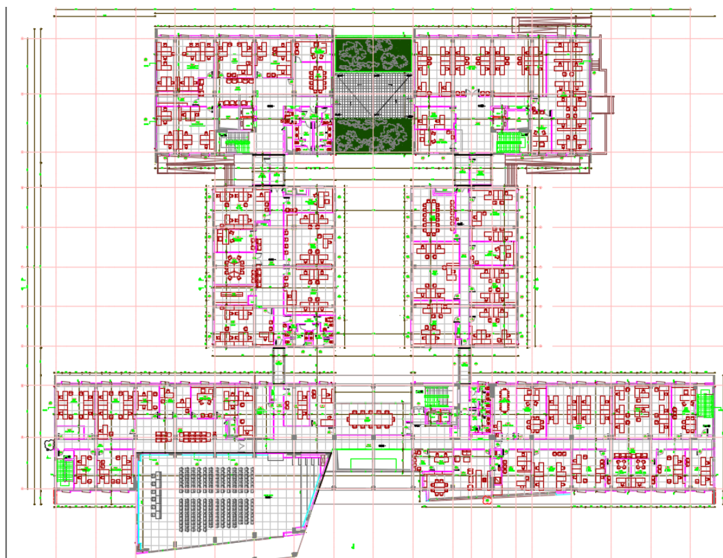
Εικόνα 14 Κάτοψη ορόφου
