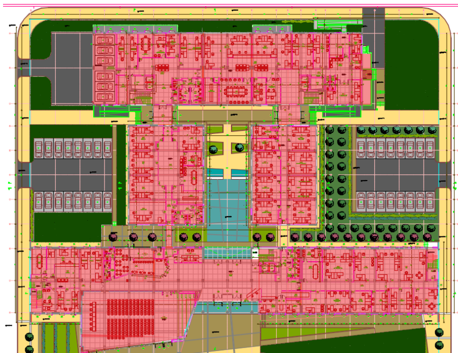
Εικόνα 53 Θερμαινόμενοι χώροι (ισόγειο)
