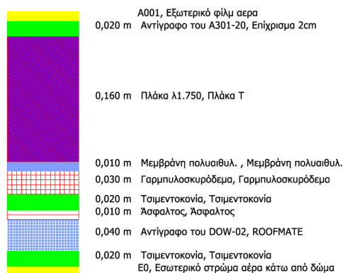
Τομή δομικού στοιχείου
