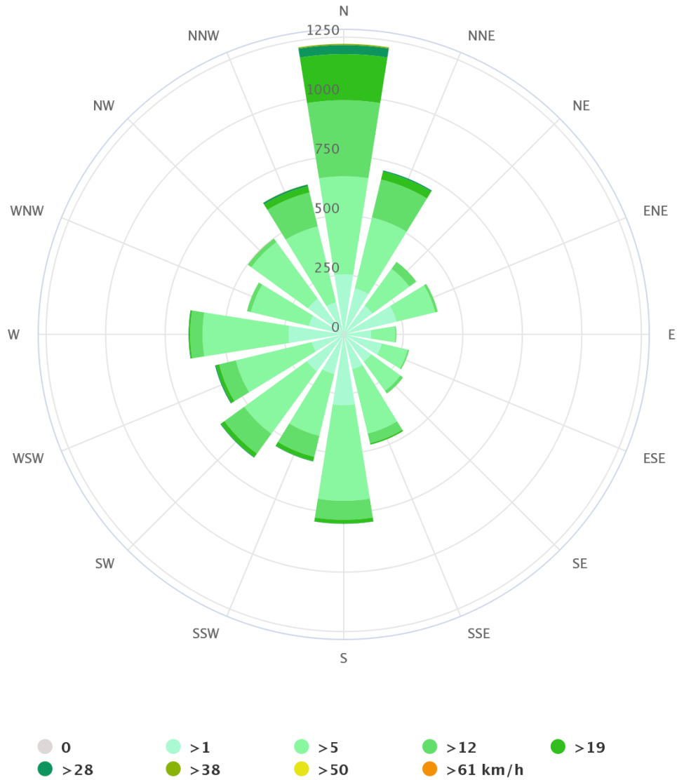
Εικόνα 61 Ανεμολόγιο
