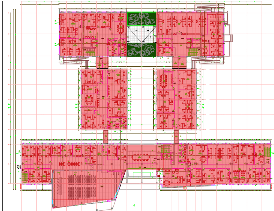
Εικόνα 52 Θερμαινόμενοι χώροι (όροφος)
