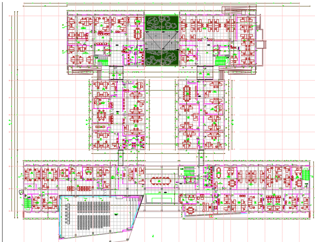
Εικόνα 14 Κάτοψη ορόφου
