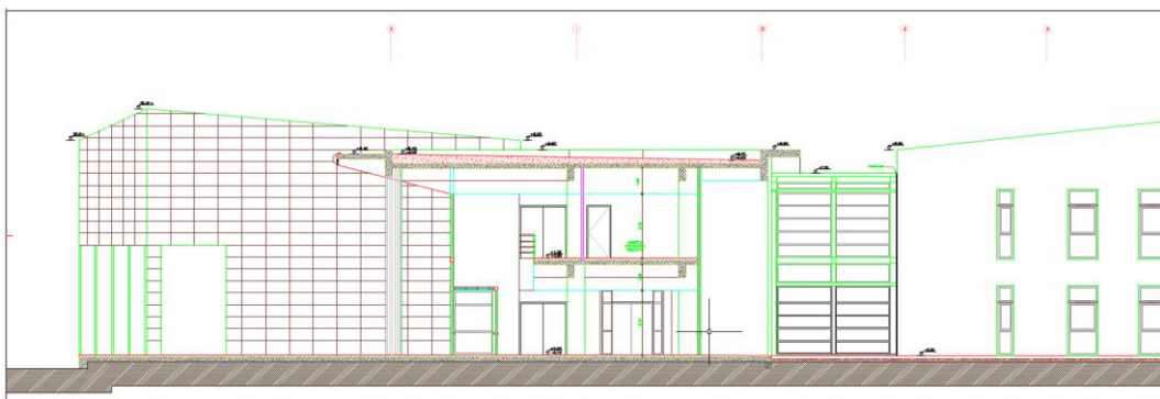
Εικόνα 30 τομή Ε-Ε τμήμα 1
