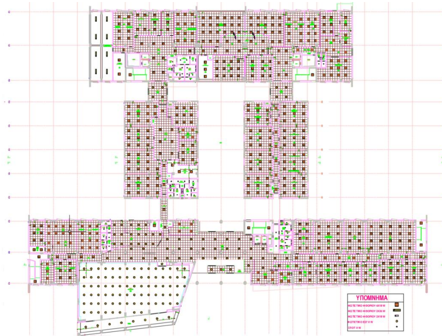
Εικόνα 76 Φωτισμός ισογείου
