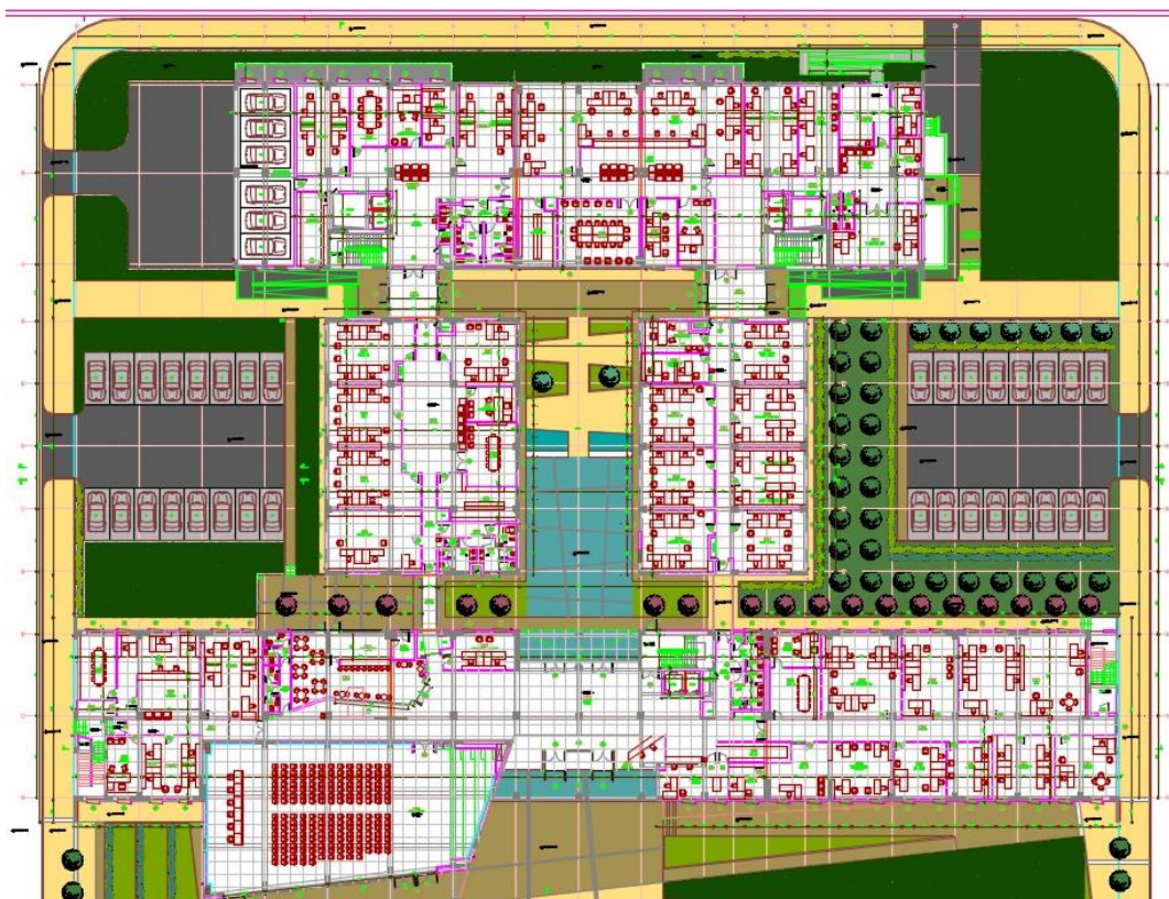
Εικόνα 13 Κάτοψη ισογείου
