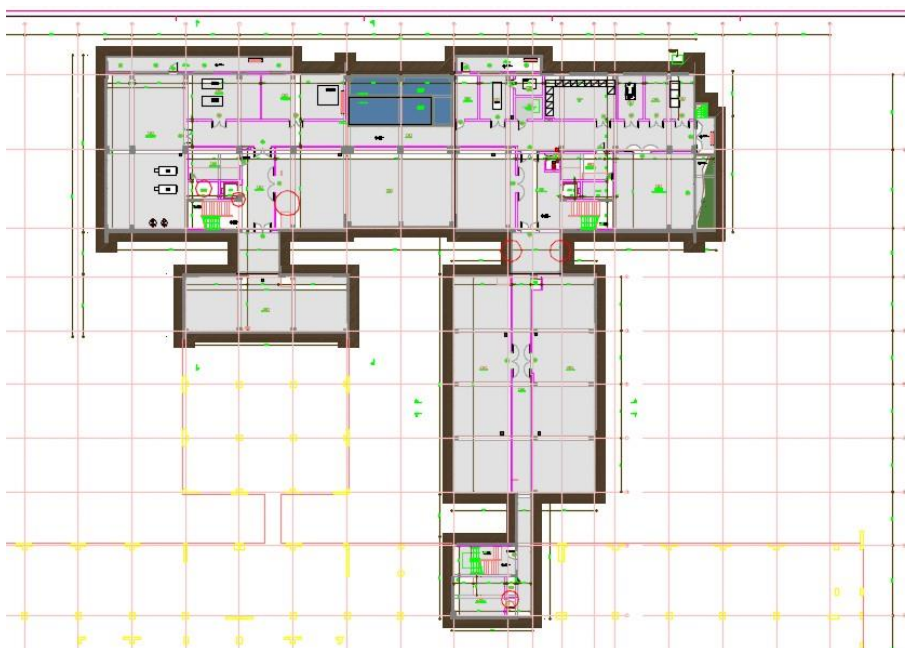
Εικόνα 54 Μη-θερμαινόμενοι χώροι (υπόγειο)
