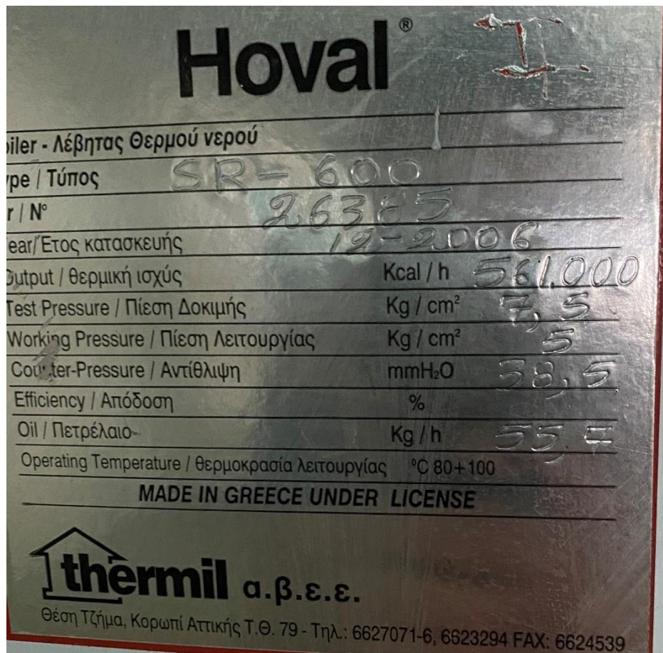
Εικόνα 64 Τα στοιχεία του λέβητα
