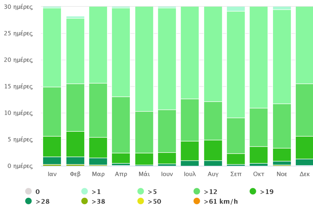
Εικόνα 60 Ταχύτητα ανέμου
