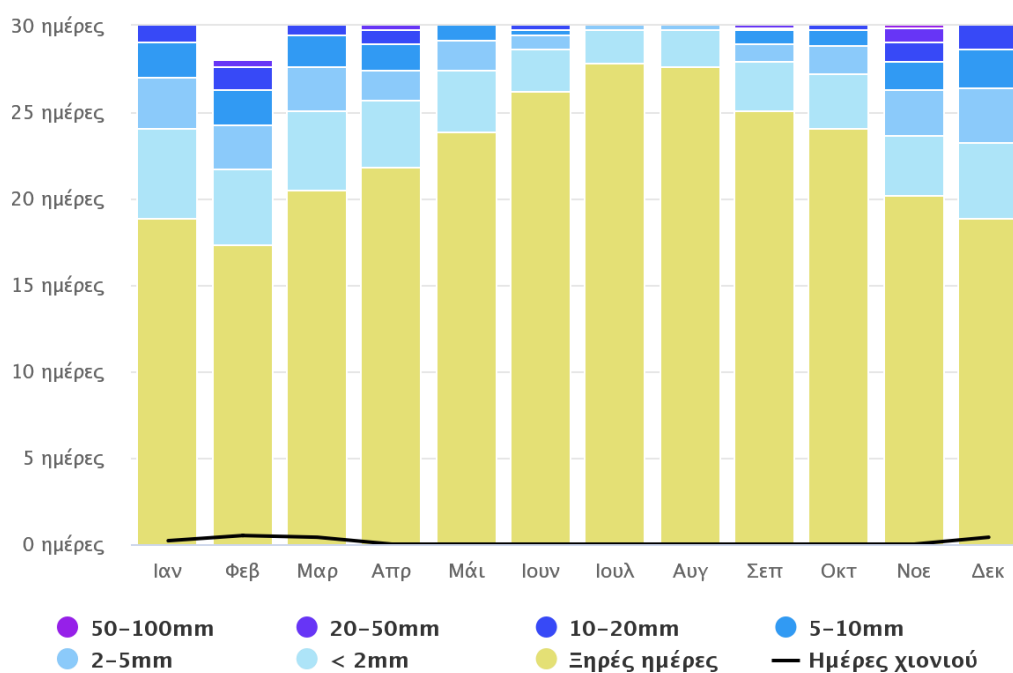
Εικόνα 59 Ποσά υετού
