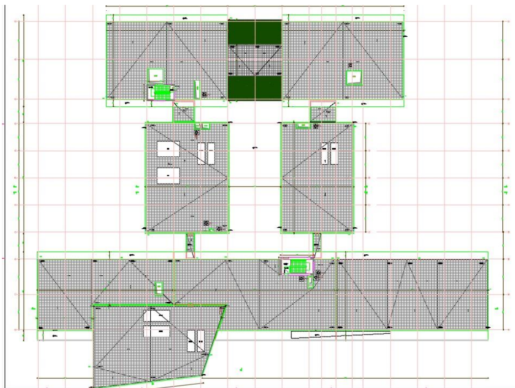
Εικόνα 15 Κάτοψη δώματος
