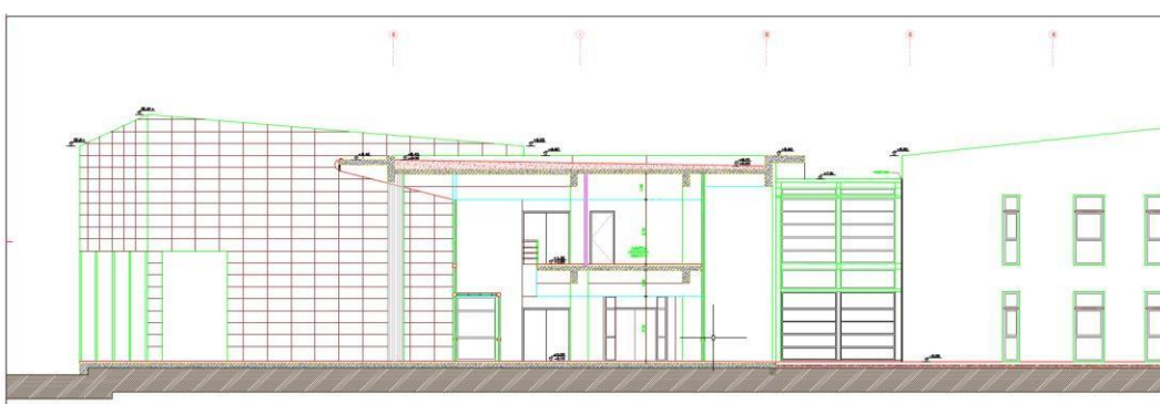
Εικόνα 30 τομή Ε-Ε τμήμα 1
