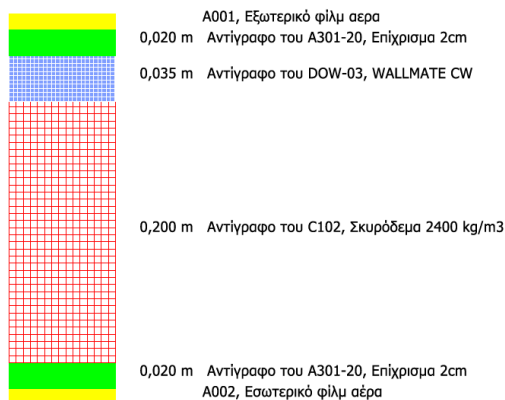
Τομή δομικού στοιχείου
