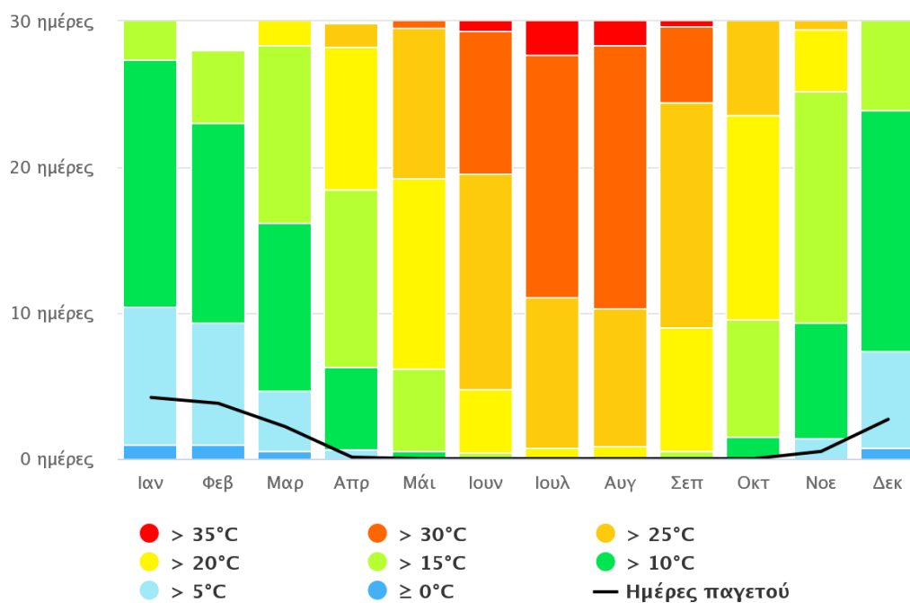
Εικόνα 58 Μέγιστες θερμοκρασίες
