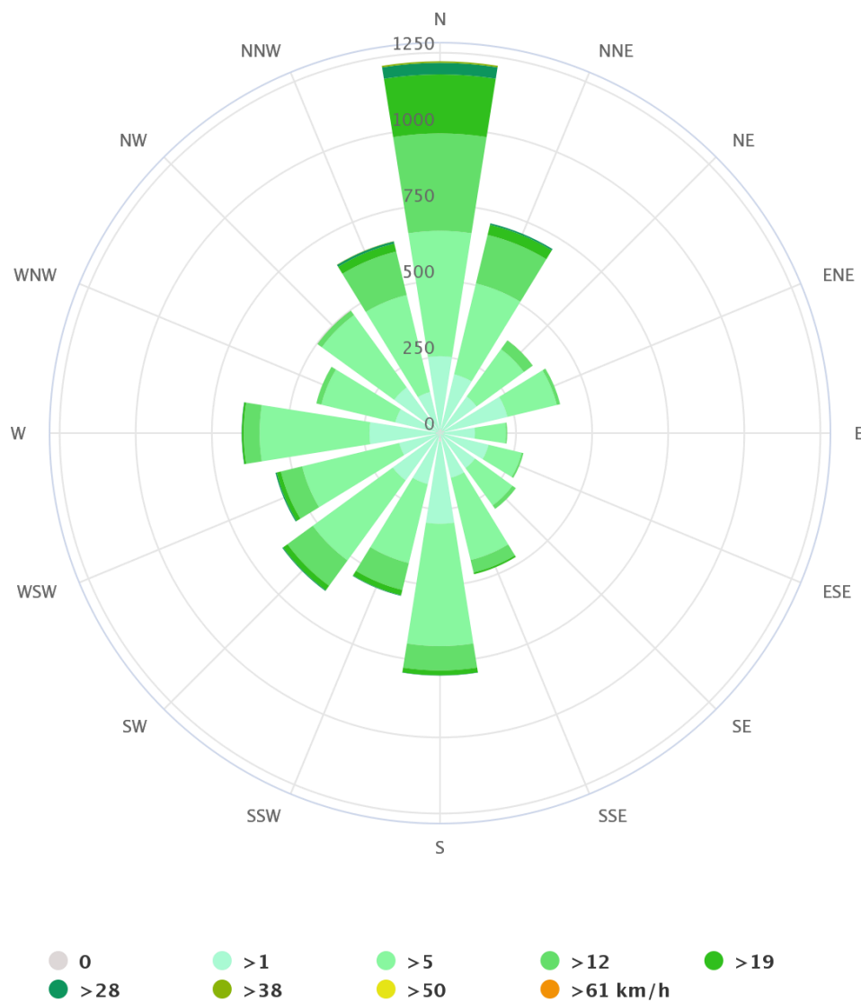
Εικόνα 61 Ανεμολόγιο
