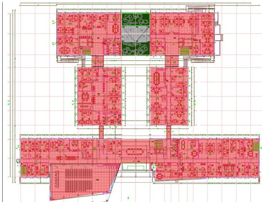
Εικόνα 52 Θερμαινόμενοι χώροι (όροφος)
