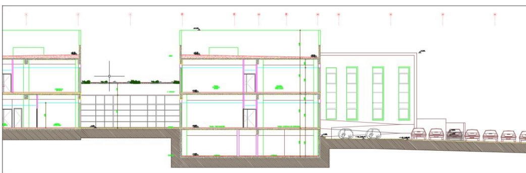
Εικόνα 27 τομή Γ-Γ τμήμα 2
