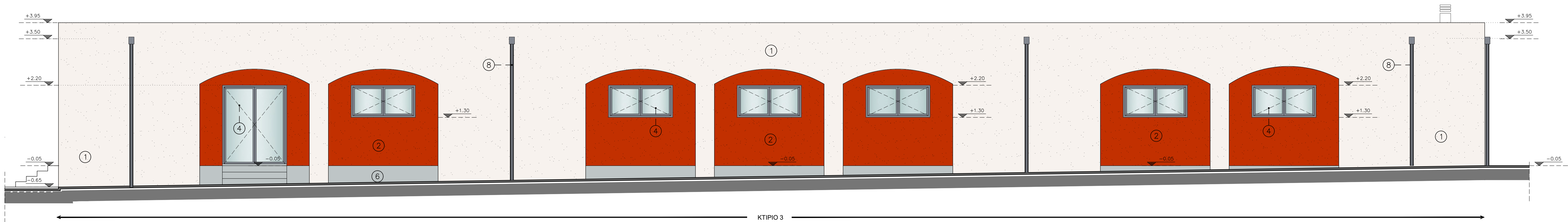
ΔΥΤΙΚΗ ΟΨΗ
