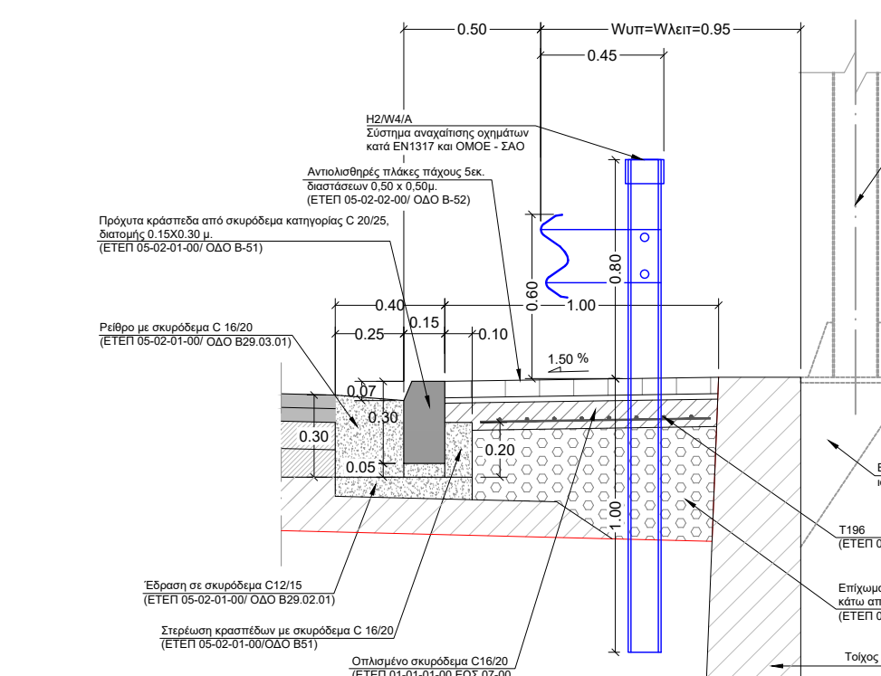
ΣΧΗΜΑ Λ4 ΛΕΠΤΟΜΕΡΕΙΑ ΠΛΕΥΡΙΚΗΣ ΔΙΑΜΟΡΦΩΣΗΣ ΑΡΤΗΡΙΑΣ ΜΕ ΠΕΖΟΔΡΟΜΙΟ ΠΛΑΤΟΥΣ 1.00, ΣΤΗΘΑΙΟ & ΤΟΙΧΟ (ΚΛΙΜΑΚΑ 1:25)
