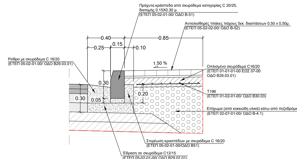
ΣΧΗΜΑ Λ1 ΛΕΠΤΟΜΕΡΕΙΑ ΠΛΕΥΡΙΚΗΣ ΔΙΑΜΟΡΦΩΣΗΣ ΑΡΤΗΡΙΑΣ ΜΕ ΠΕΖΟΔΡΟΜΙΟ ΠΛΑΤΟΥΣ 0.85 (ΚΛΙΜΑΚΑ 1:25)
