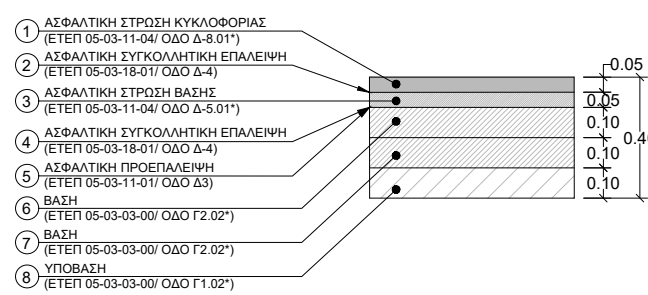
ΣΧΗΜΑ Λ9 ΛΕΠΤΟΜΕΡΕΙΑ ΔΙΑΜΟΡΦΩΣΗΣ ΟΔΟΣΤΡΩΜΑΤΟΣ ΟΔΟΥ ΠΡΟΣΒΑΣΗΣ - η2 (ΚΛΙΜΑΚΑ 1:25)
