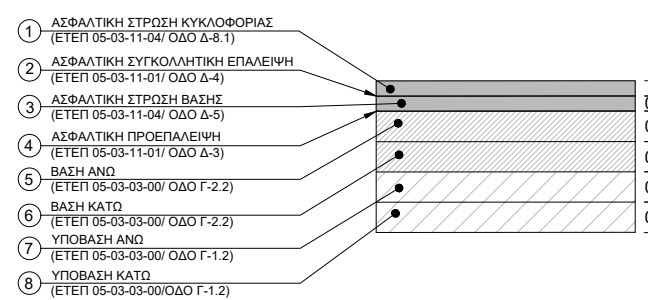
ΣΧΗΜΑ Λ7 ΛΕΠΤΟΜΕΡΕΙΑ ΔΙΑΜΟΡΦΩΣΗΣ ΟΔΟΣΤΡΩΜΑΤΟΣ ΟΔΟΥ (ΚΛΙΜΑΚΑ 1:25)
