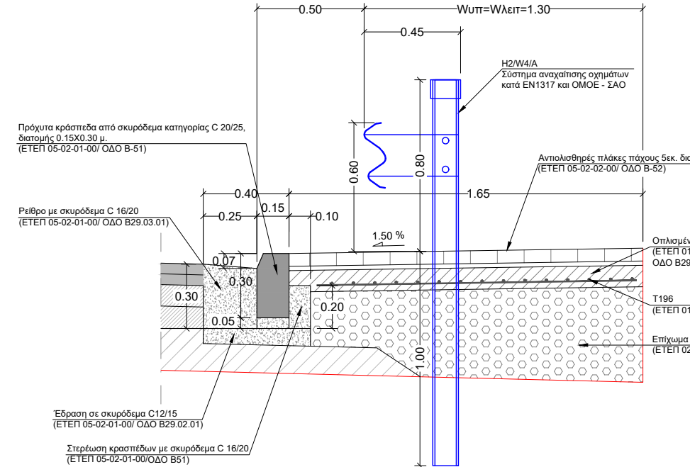
ΣΧΗΜΑ Λ3 ΛΕΠΤΟΜΕΡΕΙΑ ΠΛΕΥΡΙΚΗΣ ΔΙΑΜΟΡΦΩΣΗΣ ΑΡΤΗΡΙΑΣ ΜΕ ΠΕΖΟΔΡΟΜΙΟ ΠΛΑΤΟΥΣ 1.65 & ΣΤΗΘΑΙΟ (ΚΛΙΜΑΚΑ 1:25)
