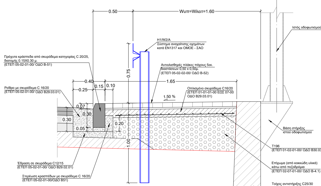
ΣΧΗΜΑ Λ5 ΛΕΠΤΟΜΕΡΕΙΑ ΠΛΕΥΡΙΚΗΣ ΔΙΑΜΟΡΦΩΣΗΣ ΑΡΤΗΡΙΑΣ ΜΕ ΠΕΖΟΔΡΟΜΙΟ ΠΛΑΤΟΥΣ 1.65, ΣΤΗΘΑΙΟ & ΤΟΙΧΟ (ΚΛΙΜΑΚΑ 1:25)
