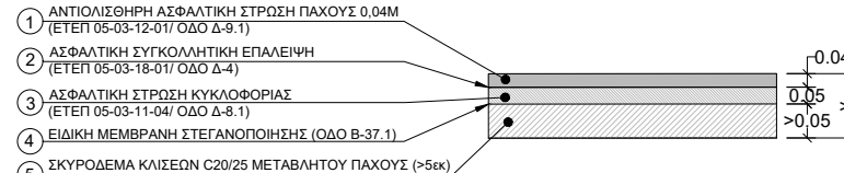
ΣΧΗΜΑ Λ8 ΛΕΠΤΟΜΕΡΕΙΑ ΔΙΑΜΟΡΦΩΣΗΣ ΟΔΟΣΤΡΩΜΑΤΟΣ ΟΔΟΥ ΚΑΤΑΣΤΡΩΜΑ ΓΕΦΥΡΑΣ (ΚΛΙΜΑΚΑ 1:25)
