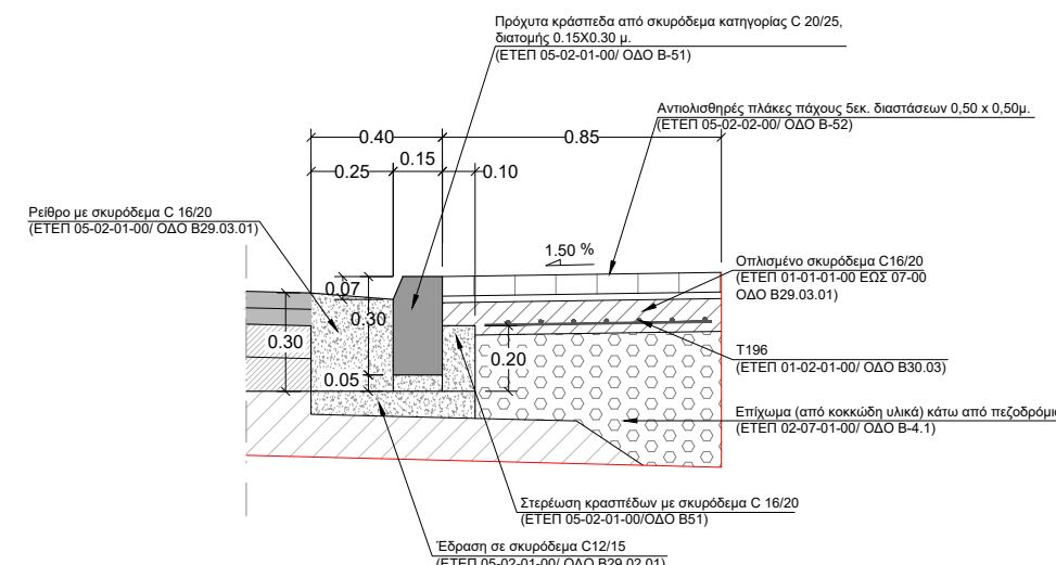
ΣΧΗΜΑ Λ2 ΛΕΠΤΟΜΕΡΕΙΑ ΠΛΕΥΡΙΚΗΣ ΔΙΑΜΟΡΦΩΣΗΣ ΑΡΤΗΡΙΑΣ ΜΕ ΠΕΖΟΔΡΟΜΙΟ ΠΛΑΤΟΥΣ 1.00 (ΚΛΙΜΑΚΑ 1:25)
