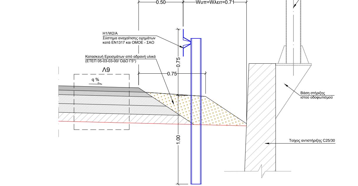
ΣΧΗΜΑ Λ6 ΛΕΠΤΟΜΕΡΕΙΑ ΠΛΕΥΡΙΚΗΣ ΔΙΑΜΟΡΦΩΣΗΣ ΑΡΤΗΡΙΑΣ ΜΕ ΕΡΕΙΣΜΑ ΠΛΑΤΟΥΣ 0.75 & ΤΟΙΧΟ (ΚΛΙΜΑΚΑ 1:25)
