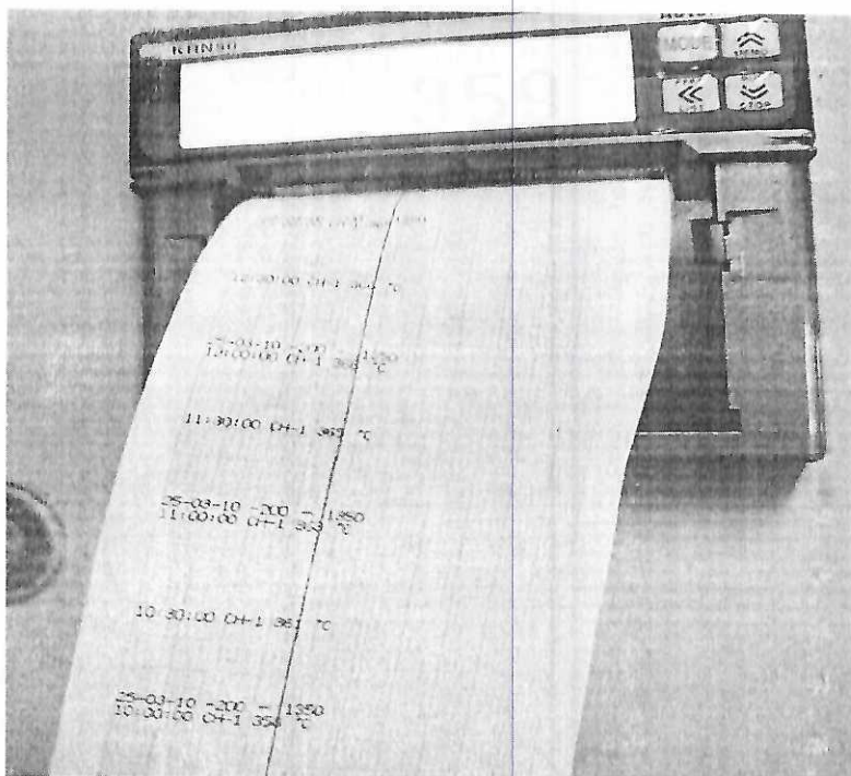
Καταγραφικό με τις ενδείξεις των θερμοκρασιών εισόδου στο 1 ο ξηραντήριο.
