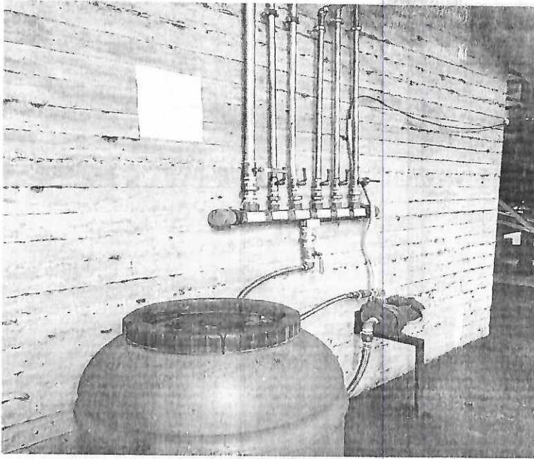
Σύστημα έγχυσης αντιοσμωτικών ουσιών στα ξηραντήρια.
